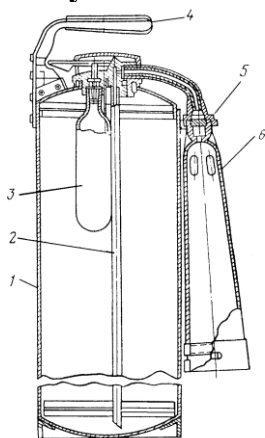
Рисунок 2. - Воздушно-пенный огнетушитель ОВП – 10
