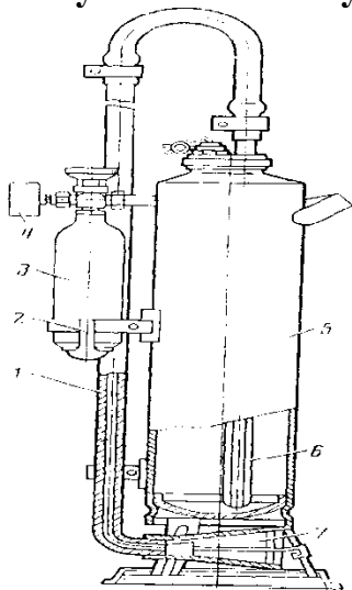
Рисунок 4 - Огнетушитель порошковый ОП – 10
