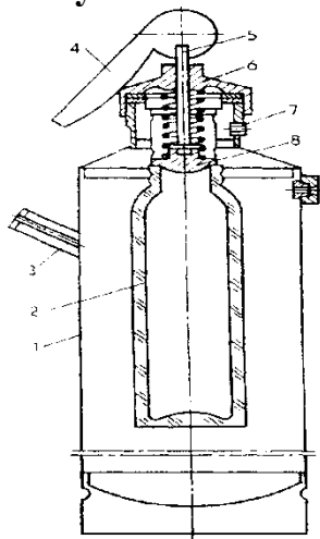
Рисунок 1. Химический пенный огнетушитель ОХП – 10
