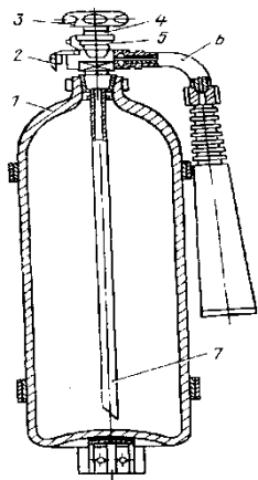
Рисунок 3 - Углекислотный огнетушитель ОУ– 5
