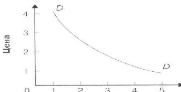
Рисунок 1 - Кривая спроса
