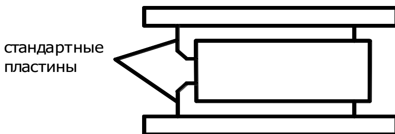
Рис.3.4. Схема испытания образцов - балочек на сжатие
