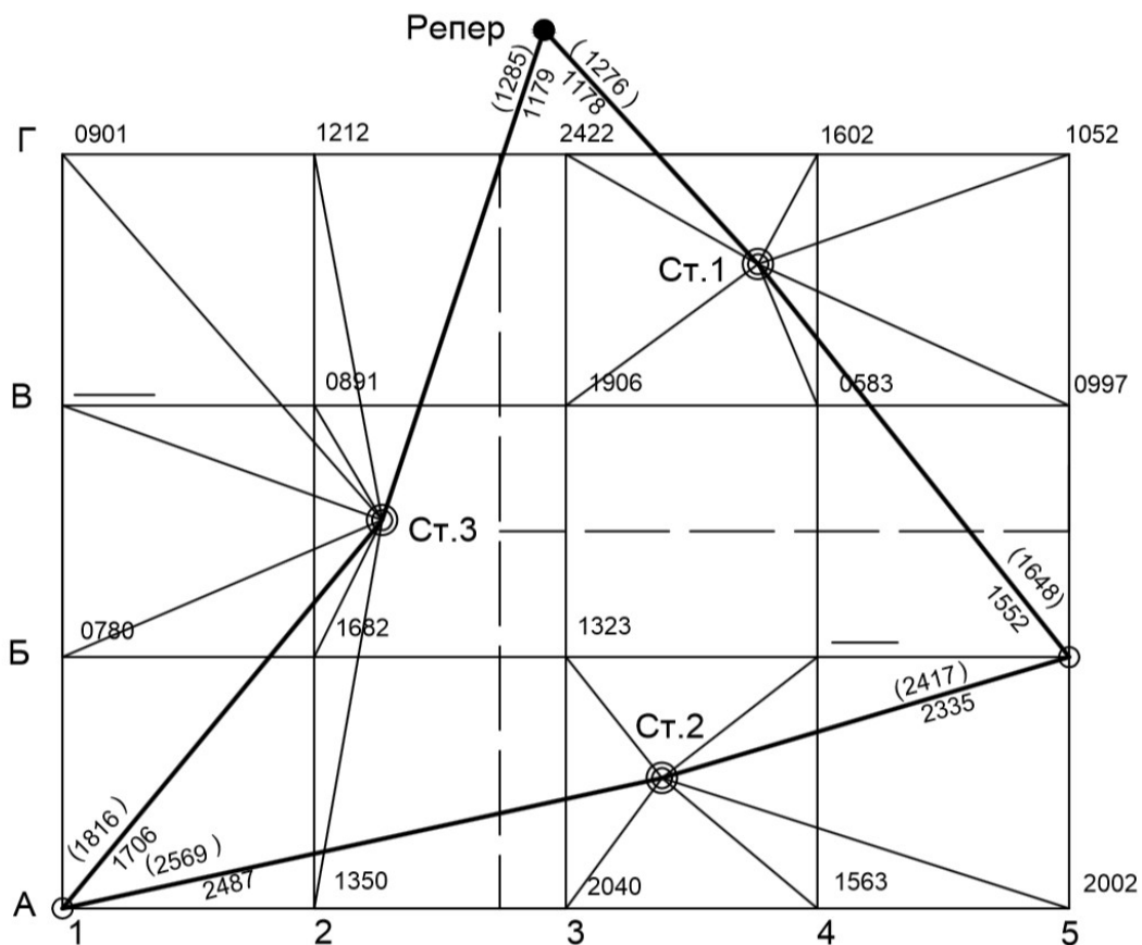
Схема нивелирования поверхности по квадратам
