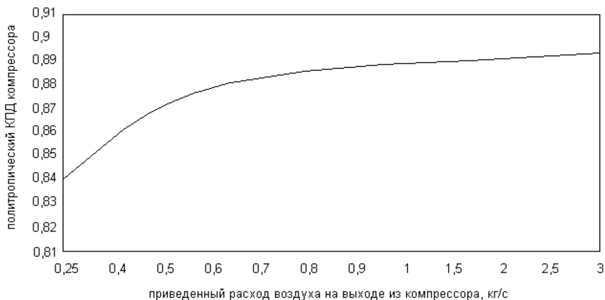
Рисунок 1. Зависимость политропического КПД осецентробежного компрессора от приведенного расхода воздуха на выходе из двигателя
