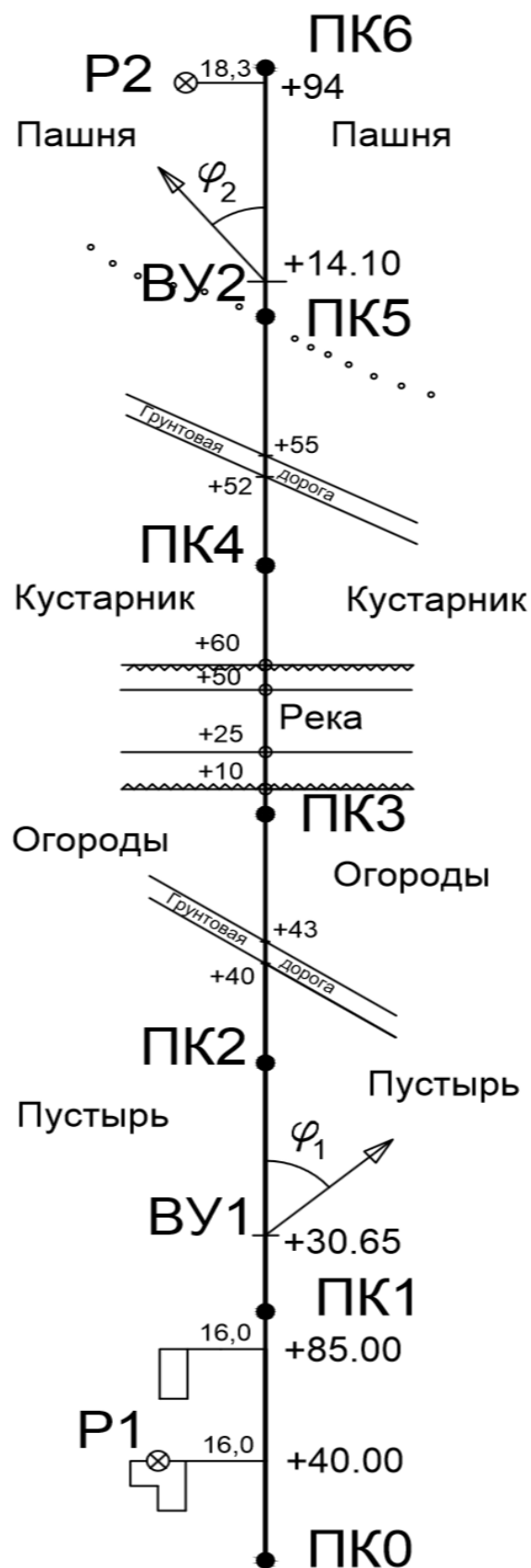
2. Пикетажный журнал
