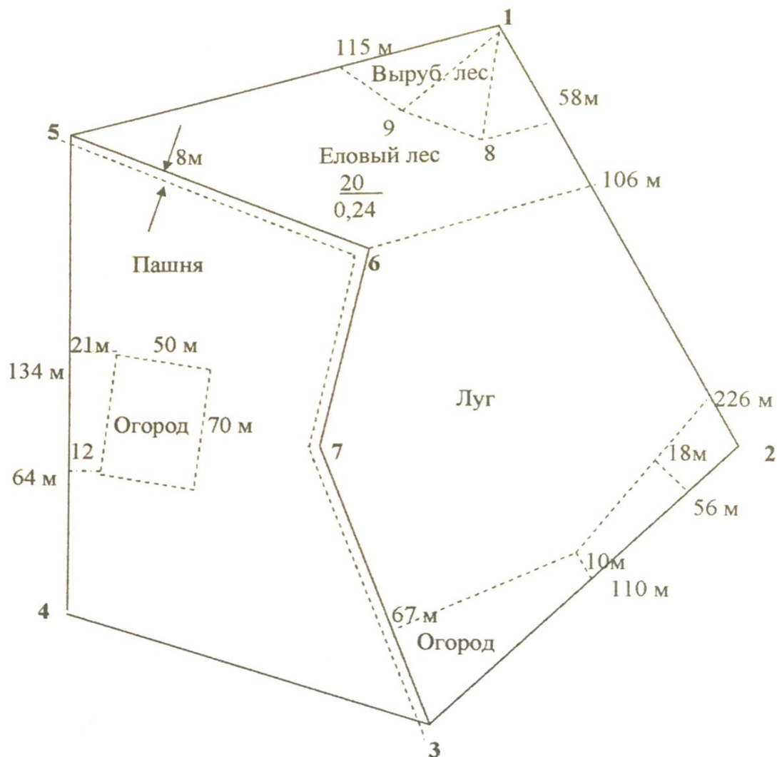
Съемка с точки 6
