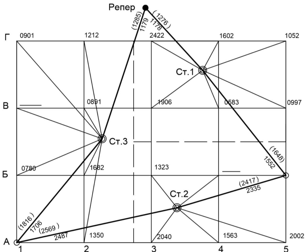
Схема нивелирования поверхности по квадратам
