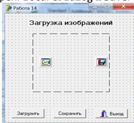
Рис. 7. Окно приложения на стадии проекта
