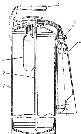
Воздушно-пенный огнетушитель ОВП – 10
