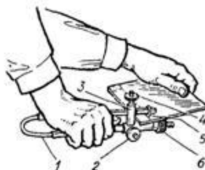
Рис. 9. Приемы резки керамических плиток с помощью роликового плиткореза: 1 - стальная пластинчатая пружина, 2 - винт-фиксатор, 3 - направляющий уголок, 4 - регулировочный винт, 5 - резец, 6 - резиновый ролик
