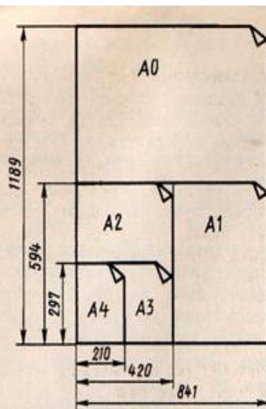
Рис. 1. Схема построения форматов
